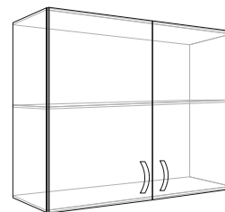
Шафа 80 В ш800*г304*в570
