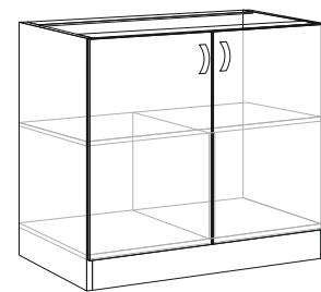
Стіл 100 Н ш1000*г464*в817
