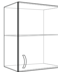
Шафа 50 В ш500*г304*в570
