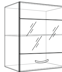
Шафа 50 ВВ ш500*г304*в570
