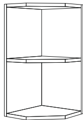
Шафа 30 ВКЗ ш280*г288*в570
