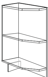
Стіл 30 НКЗ ш280*г546*в817
